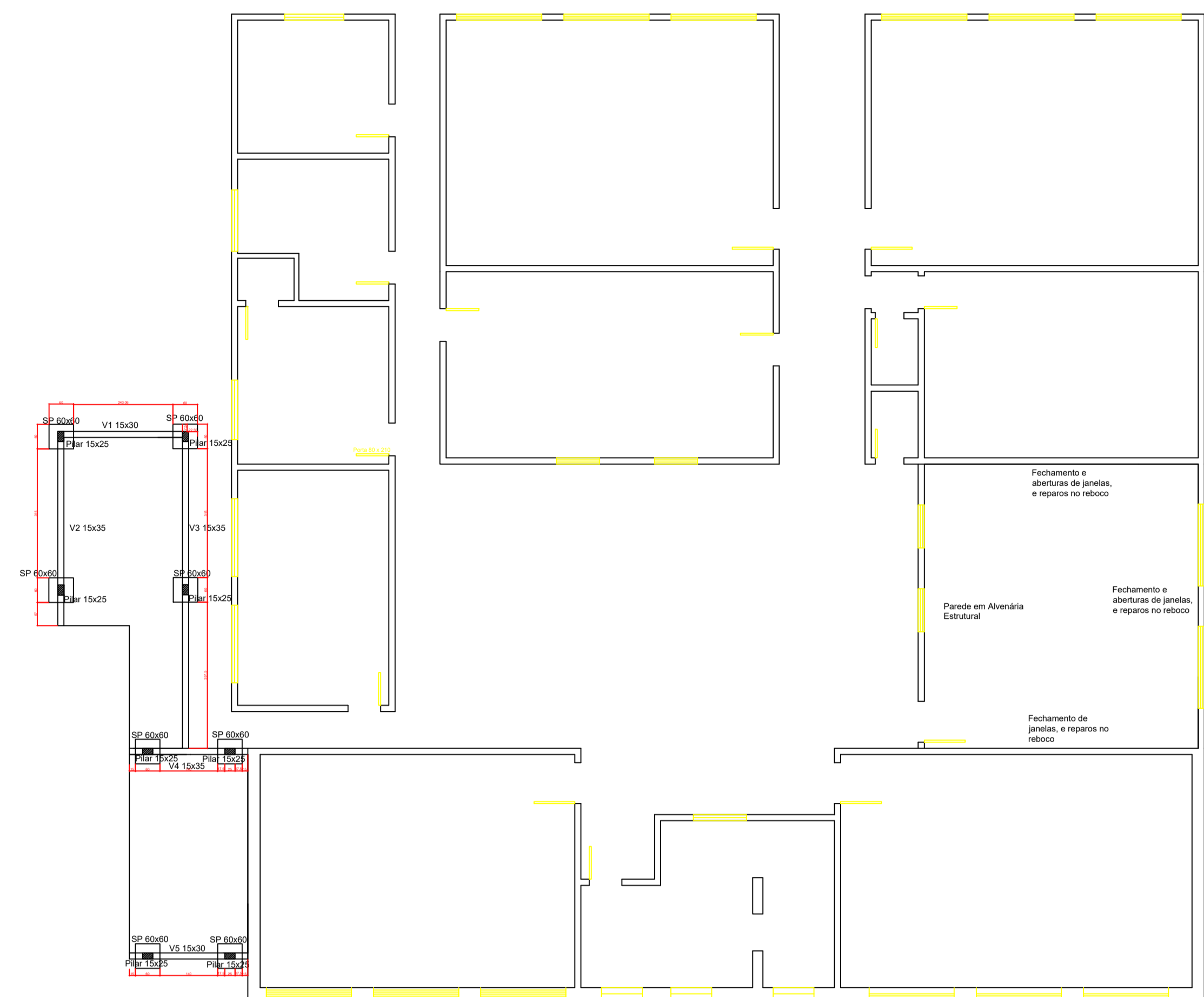
PLANTA BAIXA - LOCAÇÃO DAS SAPATAS E PILARES Esc: 1/100
