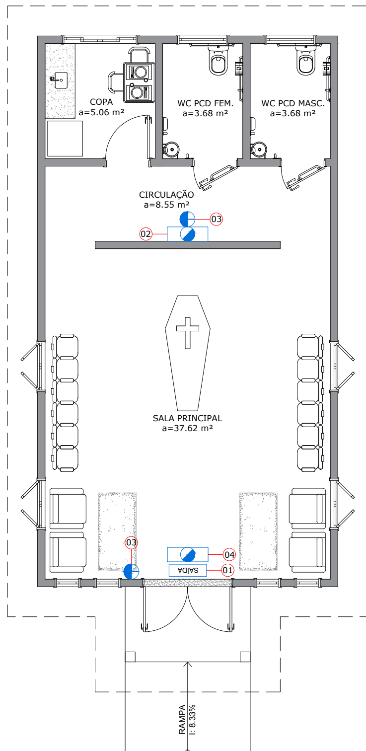
1 PLANTA BAIXA RPCI-S ESCALA 1/75
