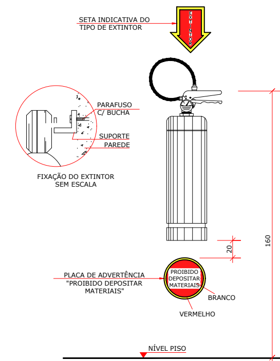
DETALHE 03: EXTINTOR DE PAREDE SEM ESCALA
